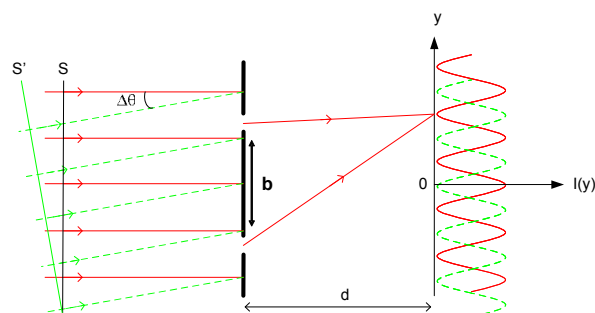
Considera-se, por simplicidade, uma análise a duas fontes pontuais no infinito separadas angularmente de \Delta\theta . Figura 6. Experiência das fendas de Young. Padrões de interferência sobrepostos, correspondentes a fontes pontuais no infinito separadas angularmente de \Delta\theta .
