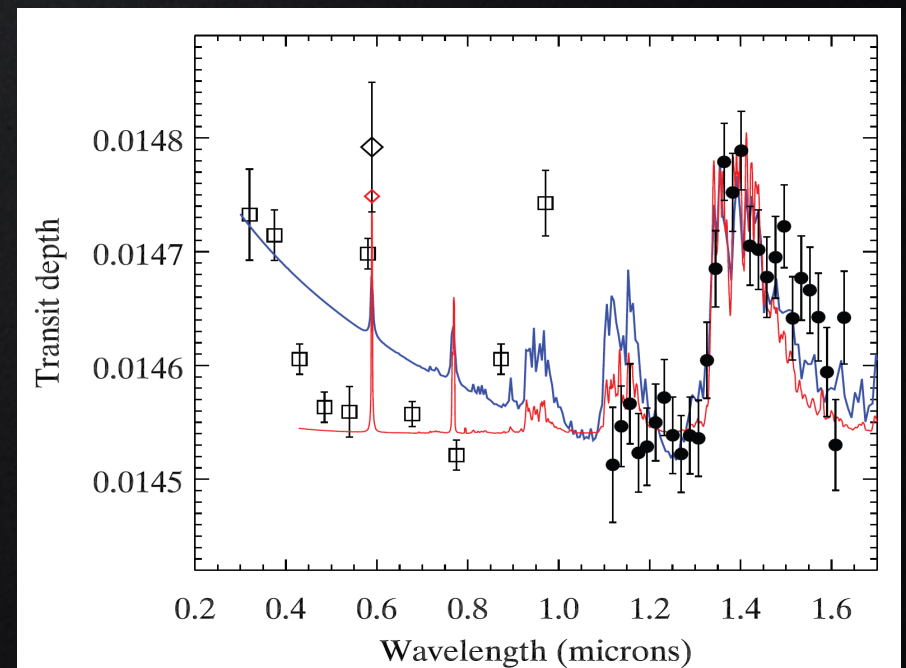
HD 209458b (Deming et al 2013)
